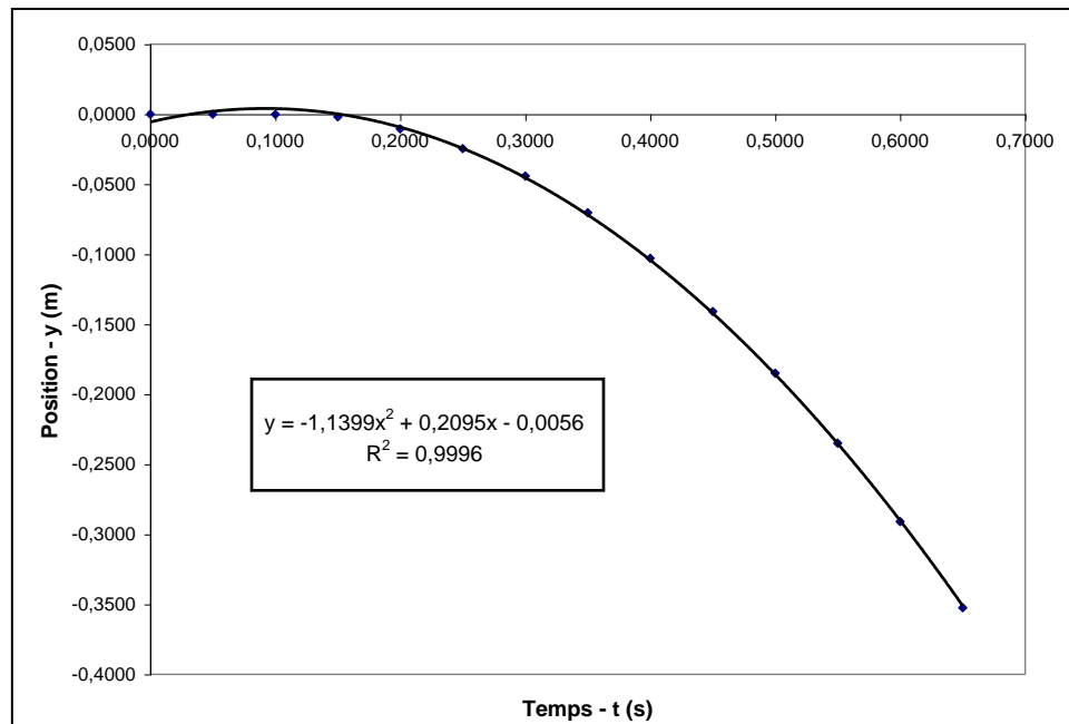
FIGURE 2. Position du mobile en fonction du temps
